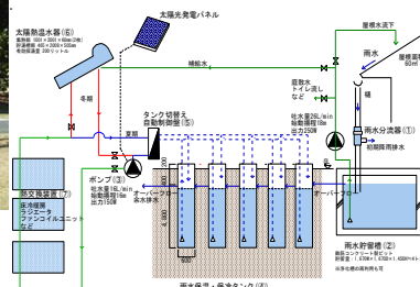
自然冷暖房システム図
