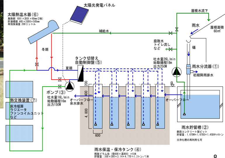
自然冷暖房システム図
